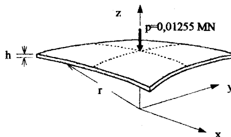
FIGURA 7 - Casca ortótropa viscoelástica
