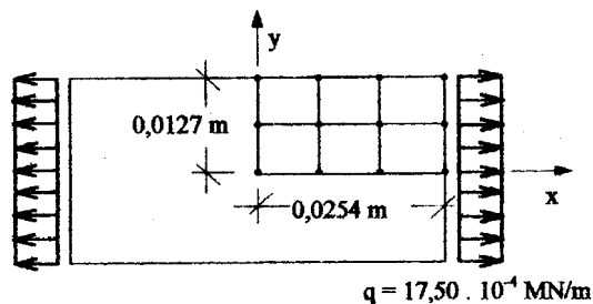
FIGURA 4 - Painel de grafite/epóxi tracionado
