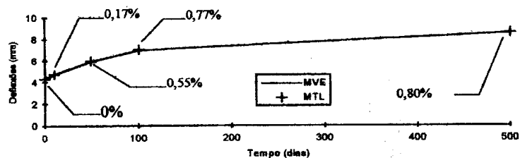
FIGURA 2 - Deflexões para o centro da laje viscoelástica
