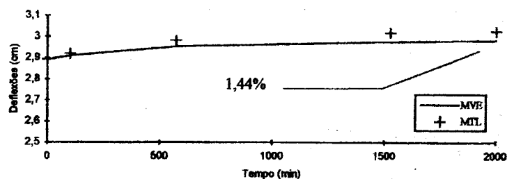
FIGURA 8 - Deflexões para o centro da casca
