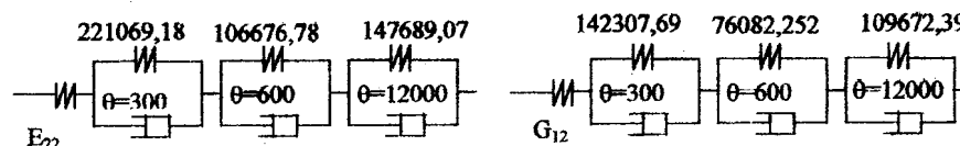
FIGURA 5 - Cadeias Kelvin nas direções 2-2 e 1-2 das lâminas
