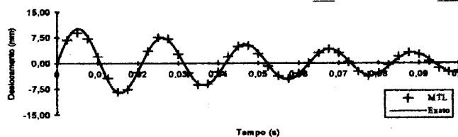
FIGURA 3 - Saída de Resultados para a colisão das placas
