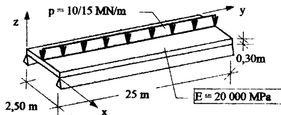
FIGURA 1 - Laje isótropa viscoelástica
