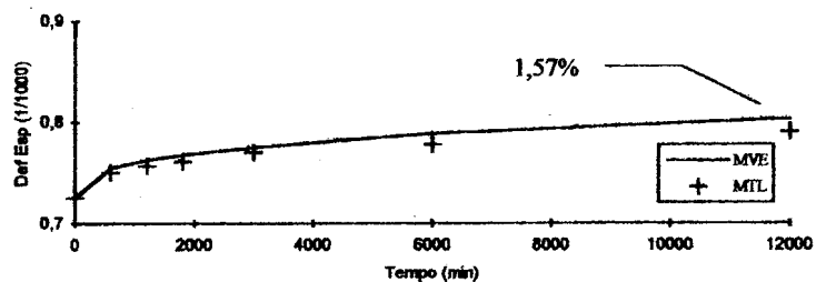
FIGURA 6 - Deformações específicas do painel
