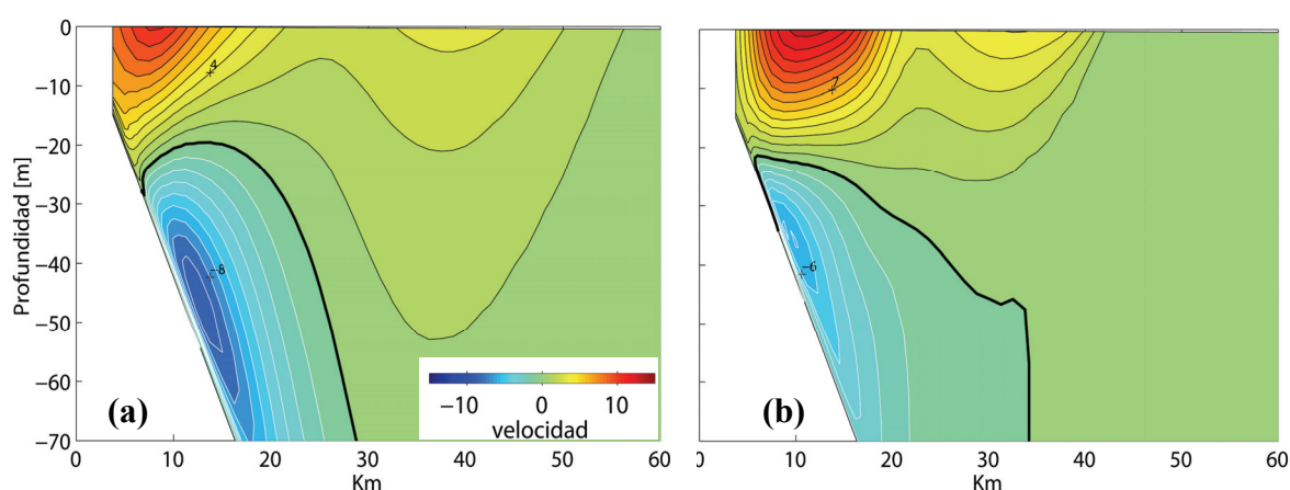
Figura 8. Comparación de la estructura de velocidad a lo largo de la costa en la sección D para el caso C10 y para los grupos de experimentos AMCBC (a) y AM0CBC (b).
