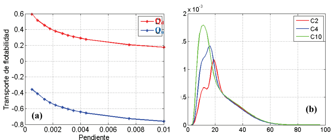
Figura 5: Comparación de los casos sin fricción (AMCBC0) para distintas pendientes. a) Transporte de flotabilidad para todas las pendientes a través de las secciones D (rojo) y U (azul) y b) Término baroclínico de presiones en la capa de fondo para C2 (verde), C4 (azul) y C10 (verde) en la sección U.
