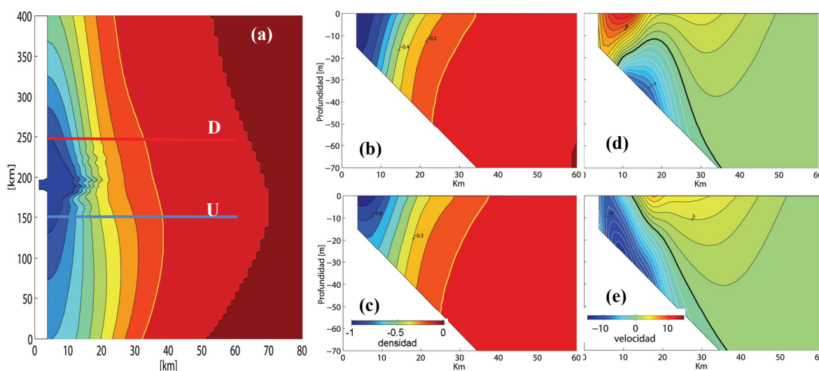
Figura 3: Caso base, AMCBC0-C4 (Día 90). (a) Densidad superficial. (La escala horizontal está aumentada para mejor visualización). La línea gruesa amarilla indica la isopícna (línea de igual densidad) de 0.1. (b) y (c) Cortes de densidad en las regiones D y U respectivamente. (d) y (e) Cortes de velocidad a lo largo de la costa en las regiones D y U.
