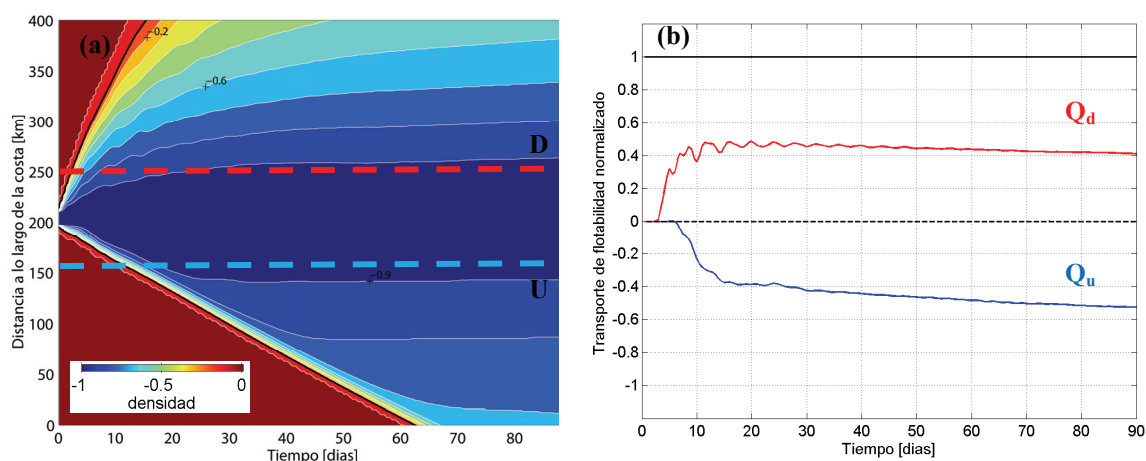
Figura 2: Caso base (AMCBC0-C4). a) Diagrama de Hovmöller de densidad. b) Transporte de flotabilidad (escalado con la descarga Q ) a través de las secciones D (rojo) y U (azul) indicadas en (a)
