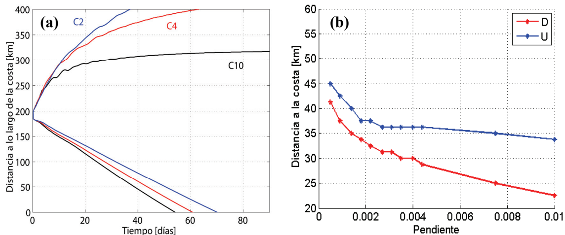
Figura 4: Comparación de los casos sin fricción de fondo (AMCBC0) para distintas pendientes. a) Diagramas de Hovmöller para la isolínea de 0.5 y para los casos C2, C4 y C10 b) Máxima expansión superficial transversal a la costa para todas las pendientes a través de las secciones D (rojo) y U (azul).
