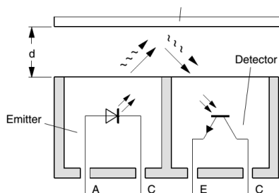
Figura 11: Disposición del LED infrarrojo y fototransistor en el interior del CNY70.
