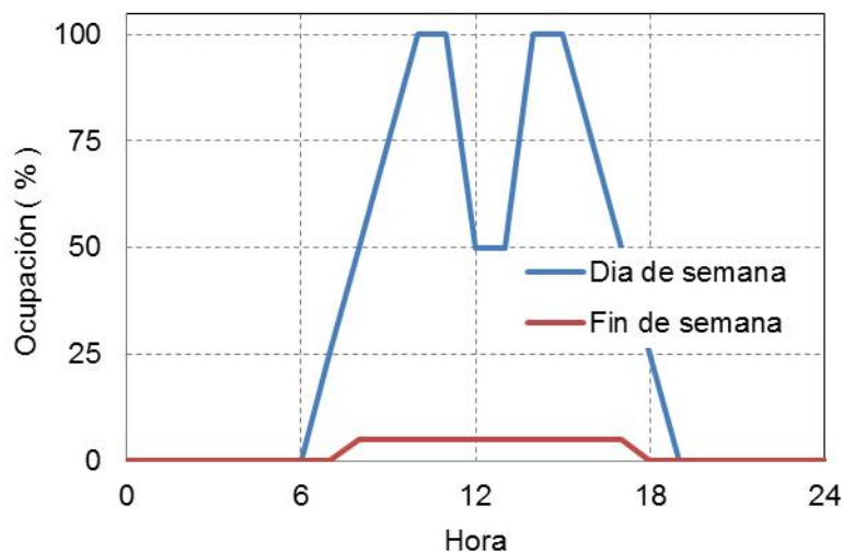
Figura 7: Modelo de ocupación del edificio de oficinas función de la hora y día de la semana
