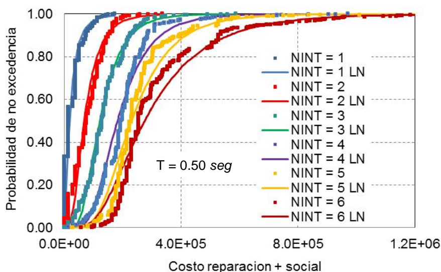
Figura 8: Costos para cada intervalo de peligrosidad sísmica. T = 0.50 seg.
