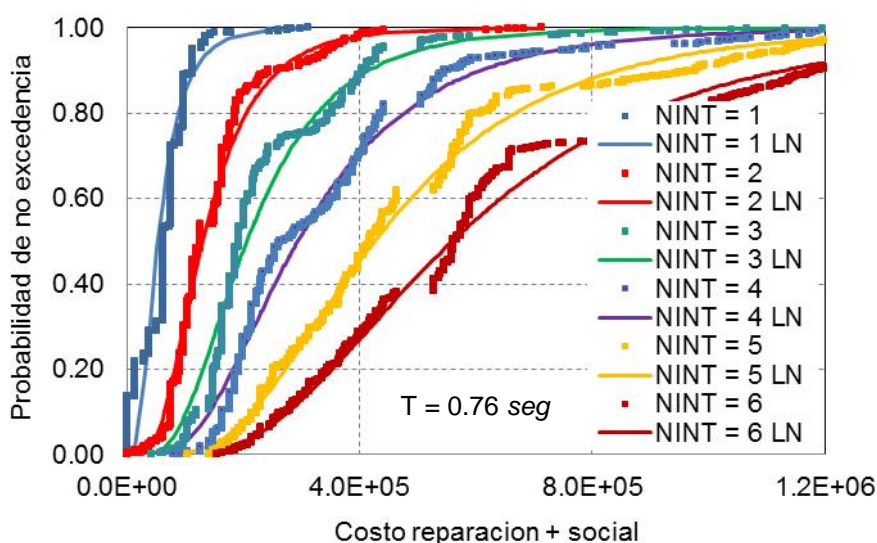
Figura 9: Costos para cada intervalo de peligrosidad sísmica. T = 0.76 seg.
