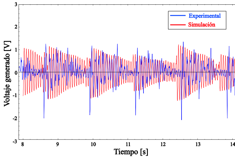
Figura 4: Respuesta temporal del voltaje generado con limite rígido (“buzzer”), \Omega = 0.8 Hz.
