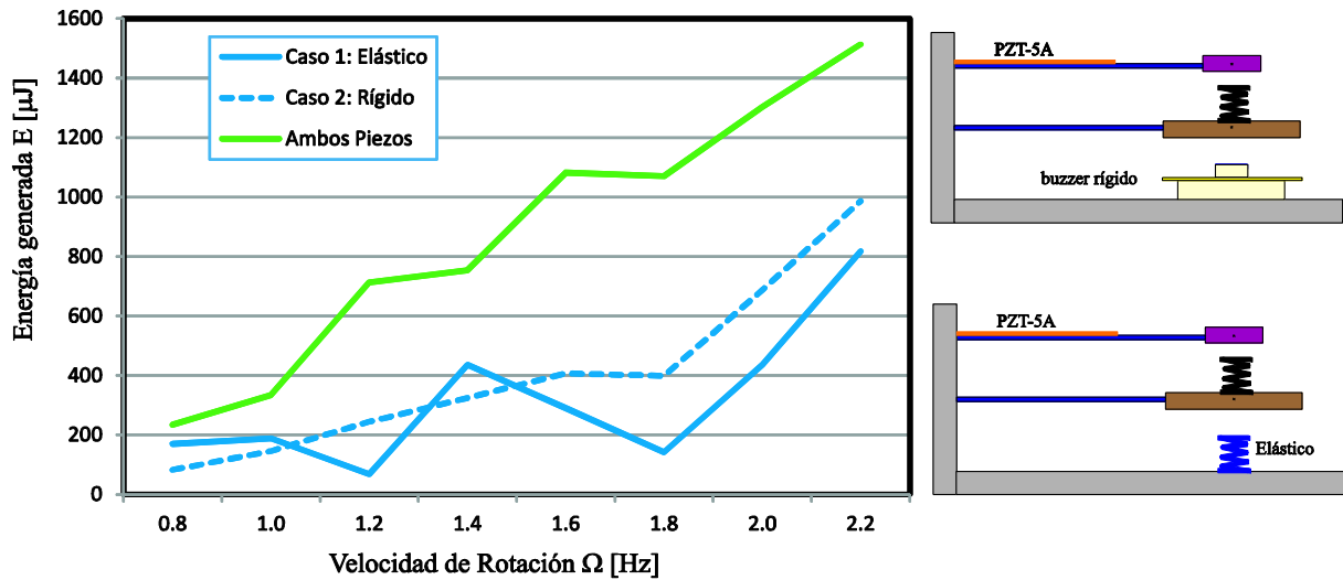
Figura 6: Energía eléctrica generada para diferentes velocidades de rotación, R = 10 \text{ k}\Omega .
