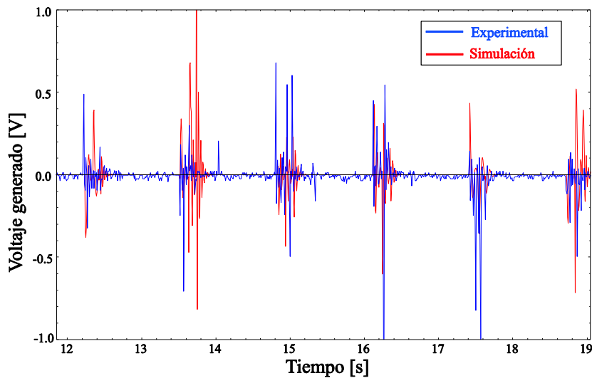
Figura 5: Respuesta temporal del voltaje generado por el “buzzer”, \Omega = 0.8 Hz.
