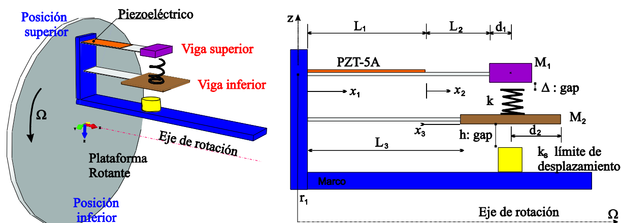
Figura 1: Esquema del dispositivo recolector.
