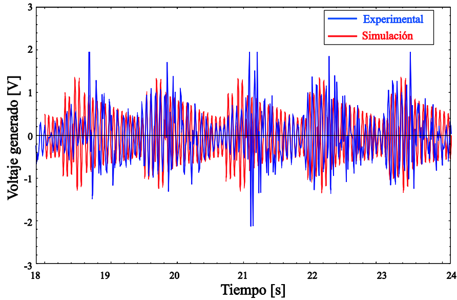
Figura 3: Respuesta temporal del voltaje generado con límite elástico, \Omega = 0.8 Hz.
